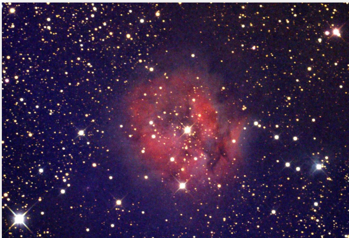
IC 5146 Nebulosa "Bozzolo" in Cygnus, Ravaldino in Monte - Forlì, 1 settembre 2021 Foto di Davide Versari
