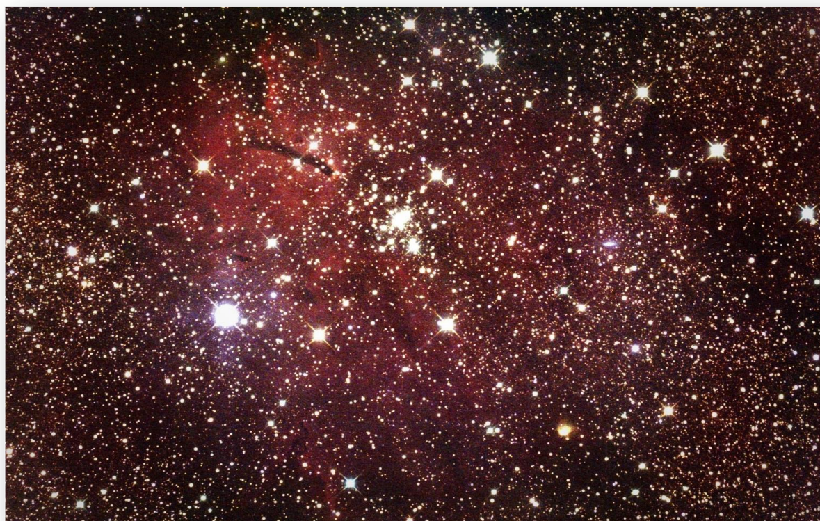
Ammasso aperto NGC 6823 in Vulpecula, Ravaldino in Monte - Forlì, 30 luglio 2021
