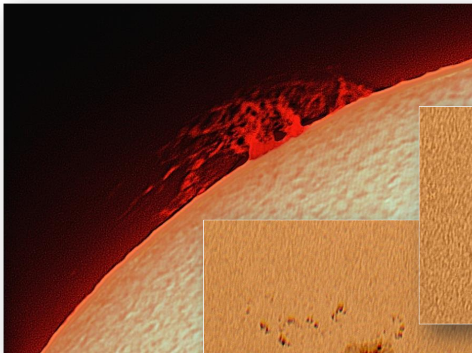
Protuberanze solari Forlì, 14 agosto 2021
